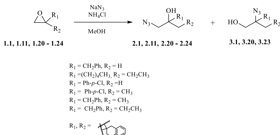
Shema 45. Priprava primarnih i sekundarnih azido alkohola 2.11 , 2.11 , 2.20 – 2.24 i 3.1 , 3.20 , 3.23
