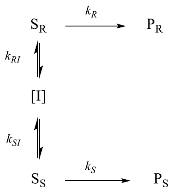
Shema 7. Enzimski katalizirana DKR 25
