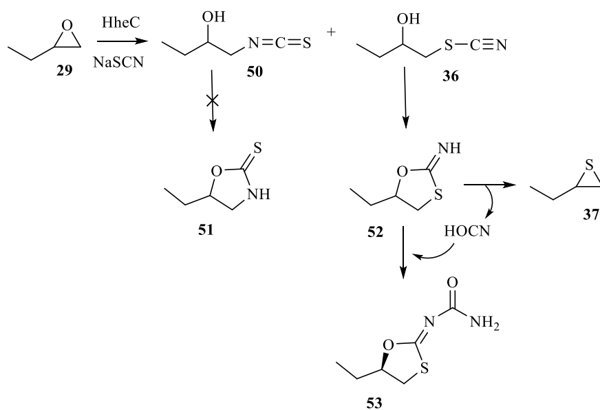
Shema 18. Mehanizam reakcije 29 s tiocijanatnim ionom
