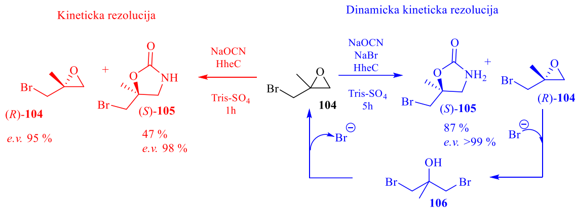
Shema 27. DKR 2-(bromometil)-2-metiloksirana ( 104 ) 8
