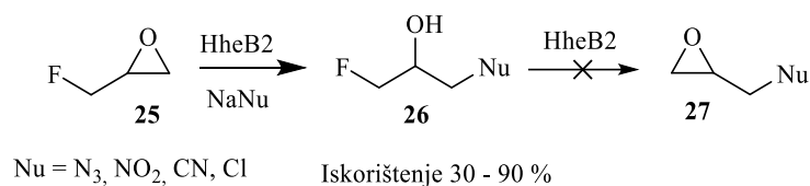
Shema 11. Reakcije 25 katalizirane HheB2 iz Mycobacterium sp. soj GP1 52
