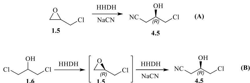
Shema 31. HHDH katalizirana sinteza 4.5 iz epiklorhidrina ( 1.5 ) (A), sinteza 4.5 iz 1,3-dikloro-2-propanola ( 1.6 ) (B)
