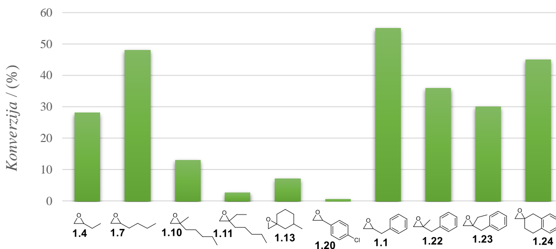
Slika 14. Aktivnost HheB prikazane prema odabranim epoksidima
