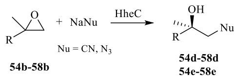
Tablica 4. Kinetička rezolucija metil-supstituiranih epoksida 54b – 58b katalizirana HheC 65
