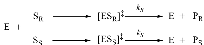
Shema 6. Enzimski katalizirana kinetička rezolucija
