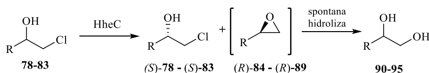
Shema 23. Kinetička rezolucija klorohidrina 78 – 83 katalizirana HheC 72
