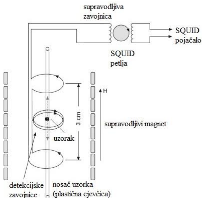
Slika 16. Pojednostavljena shema rada SQUID magnetometra [121].
