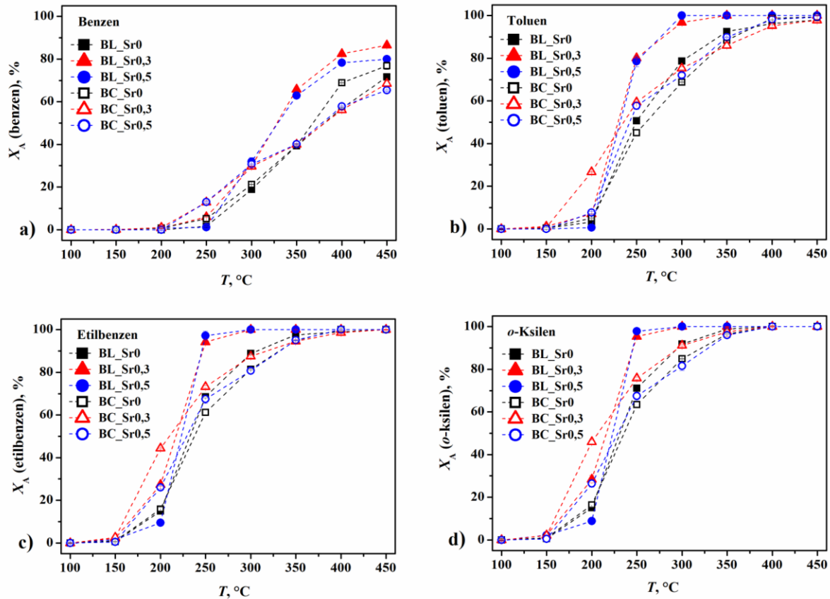
Slika 56. Prikaz konverzija (a) benzena, (b) toluena, (c) etilbenzena i (d) o -ksilena u ovisnosti o reakcijskoj temperaturi za pripremljene BSMO katalizatore.
