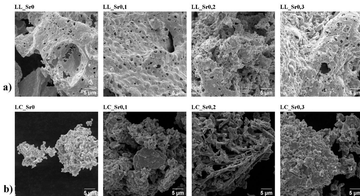
Slika 30. SEM mikrografije praškastih LSMO uzoraka pripremljenih (a) limunskim i (b) koprecipitacijskim postupkom sinteze, snimljene pri povećanju od 5000x.
