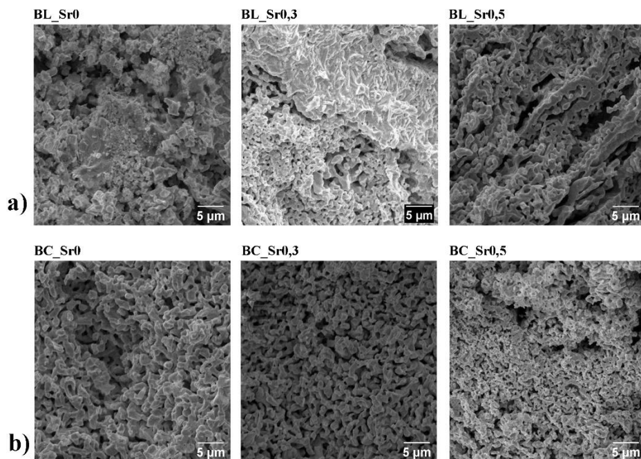
Slika 37. SEM mikrografije lomne površine BSMO peleta dobivenih iz prašaka pripremljenih (a) limunskim i (b) koprecipitacijskim postupkom sinteze, snimljene pri povećanju od 5000x.
