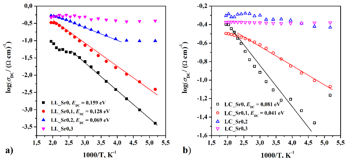
Slika 39. Arrheniusova ovisnost istosmjerne provodnosti ( \sigma_{DC} ) o recipročnoj vrijednosti temperature za LSMO uzorke pripravljene (a) limunskim i (b) koprecipitacijskim postupkom sinteze.
