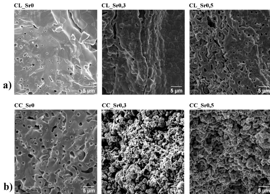
Slika 34. SEM mikrografije lomne površine CSMO peleta dobivenih iz prašaka pripremljenih (a) limunskim i (b) koprecipitacijskim postupkom sinteze, snimljene pri povećanju od 5000x.
