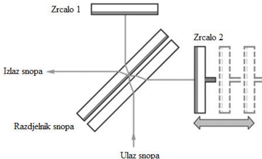
Slika 12. Shematski prikaz Michelsonovog interferometra [110].
