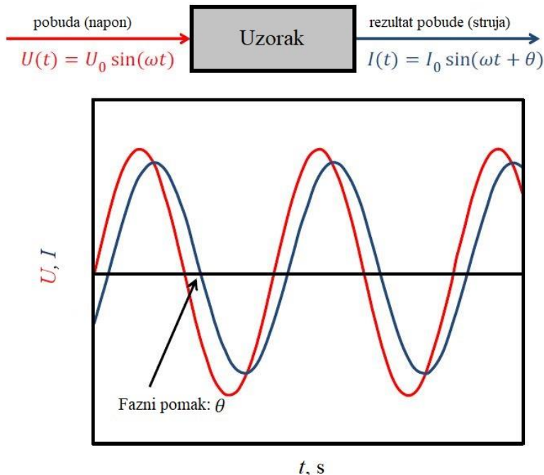
Slika 14. Osnovni princip rada impedancijske spektroskopije [117].
