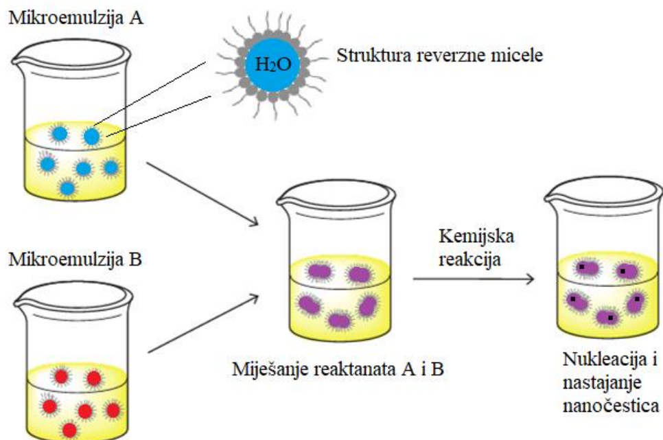
Slika 6. Shematski prikaz sinteze nanočestica postupkom reverzne mikroemulzije (prema [72]).
