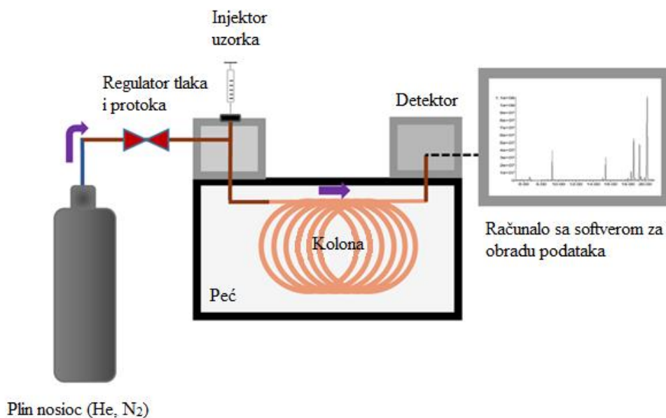
Slika 18. Shematski prikaz sustava za plinsku kromatografiju [124].
