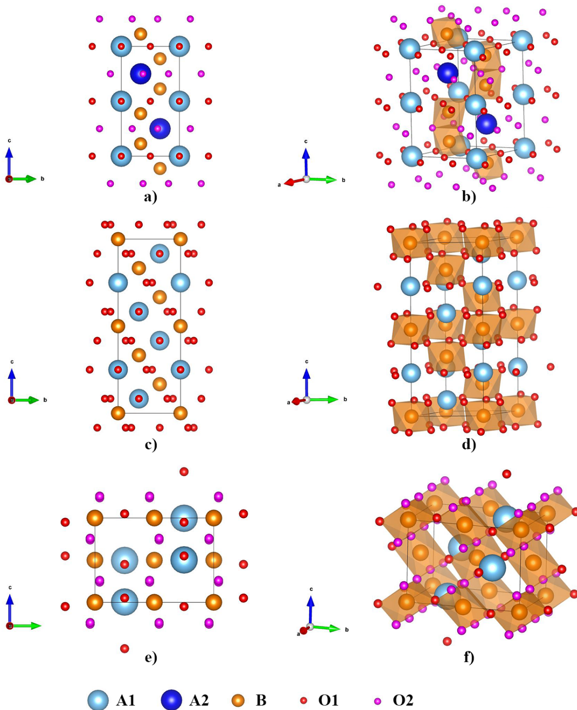
Slika 2. (a, b) P6_3/mmc i (c, d) R\bar{3}c vrste heksagonske distorzije i (e, f) Pnma ortorompska distorzija perovskitne rešetke. Kristalne strukture u smjeru osi a prikazane su pod (a, c i e), dok su trodimenzionalne sheme s označenim BO_6 oktaedrima prikazane pod (b, d i f). Prikazi struktura izrađeni su u računalnom programu VESTA 3 [21].
