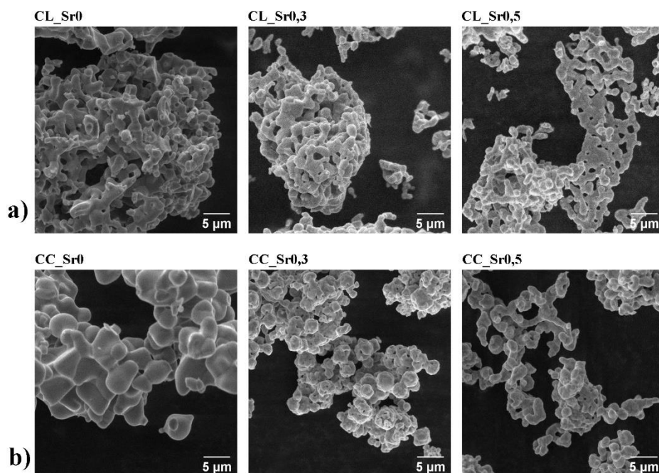
Slika 33. SEM mikrografije praškastih CSMO uzoraka pripremljenih (a) limunskim i (b) koprecipitacijskim postupkom sinteze, snimljene pri povećanju od 5000x.
