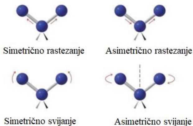
Slika 11. Vrste vibracija u molekulama (prema [109]).
