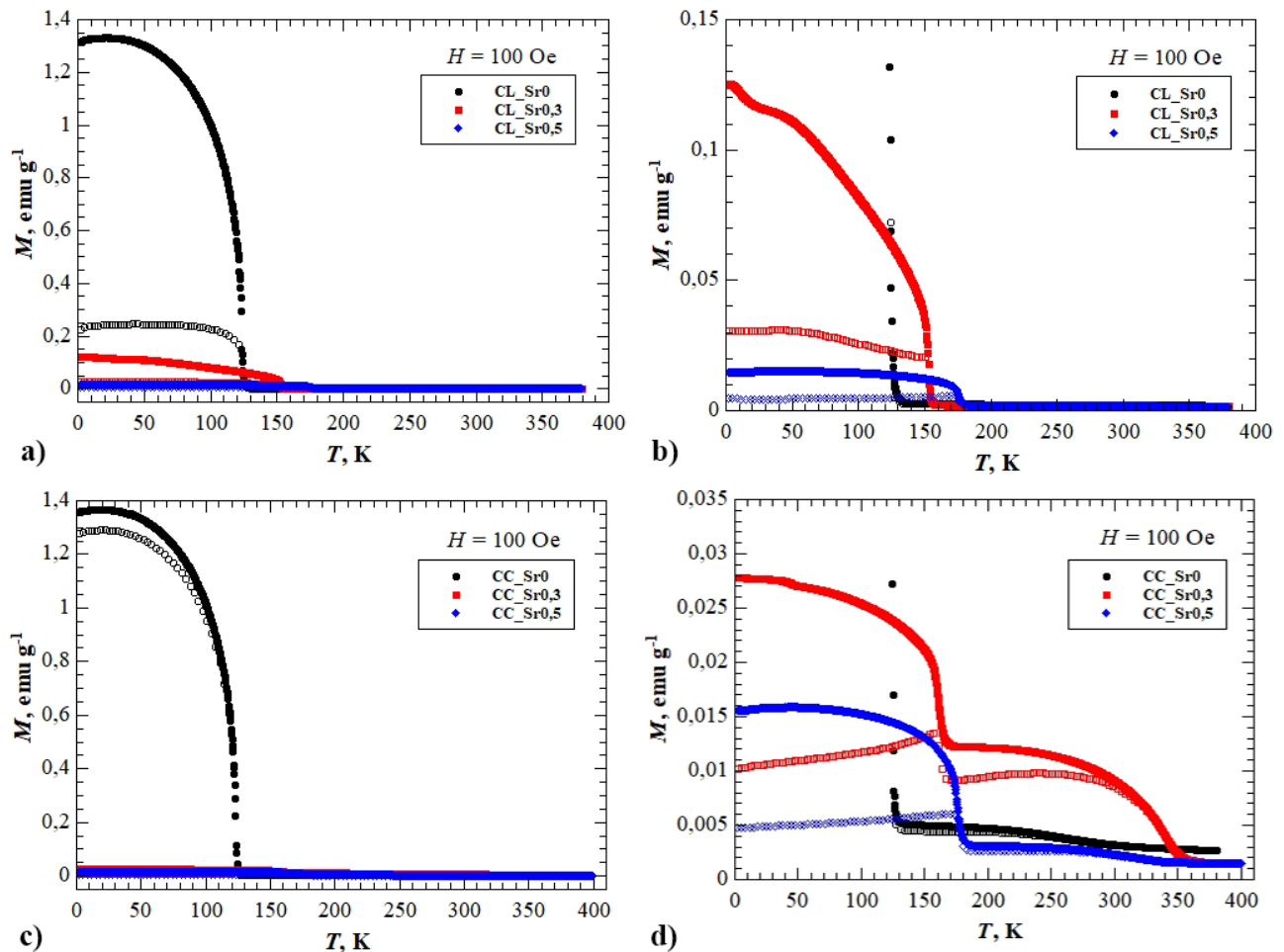
Slika 50. Magnetizacijske krivulje uzoraka CSMO pripremljenih limunskim (oznake CL, a i b) i koprecipitacijskim (oznake CC, c i d) postupkom sinteze izmjerene pri jakosti magnetskog polja od 100 Oe. Na slikama (b) i (d) dani su uvećani prikazi krivulja za dopirane uzorke. Prazni simboli predstavljaju ZFC mjerenja, a ispunjeni FC mjerenja.
