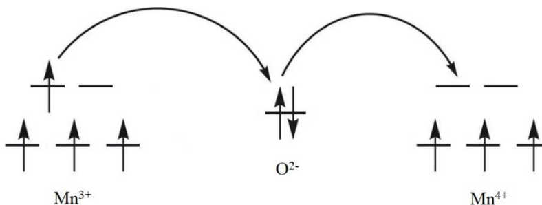
Slika 8. Shematski prikaz Zenerovog mehanizma izmjene u magnanitima.
