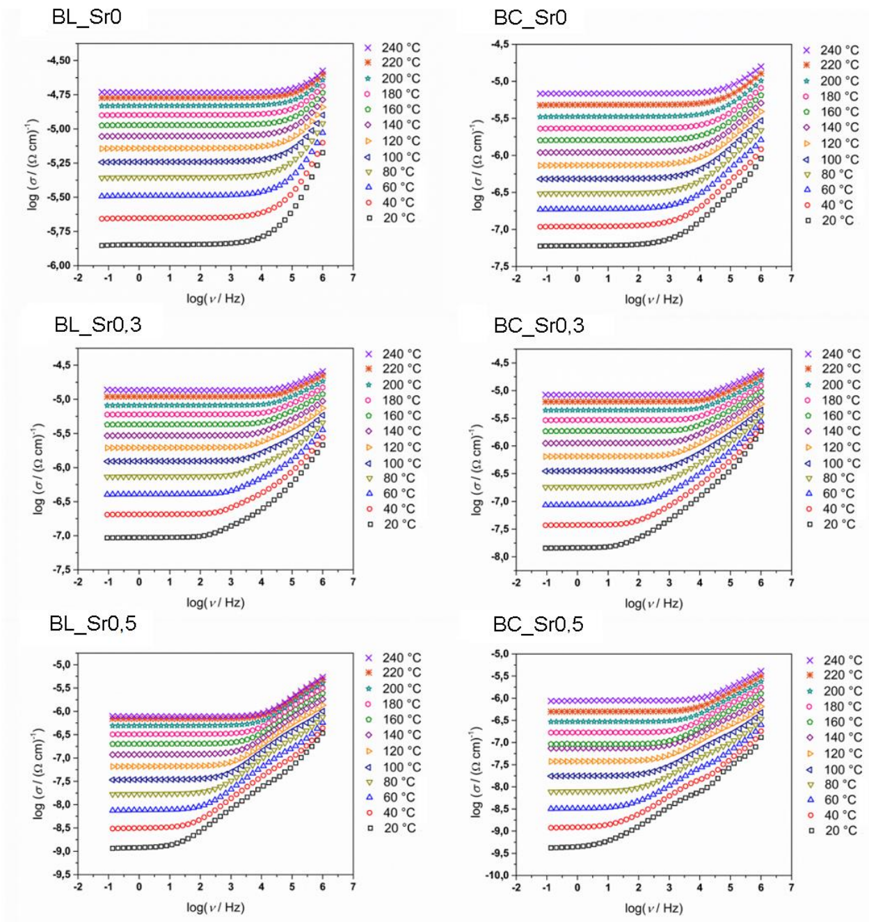
Slika P3. Frekvencijske ovisnosti električne provodnosti BSMO uzoraka pripremljenih limunskim (oznake BL) i koprecipitacijskim (oznake BC) postupkom sinteze.
