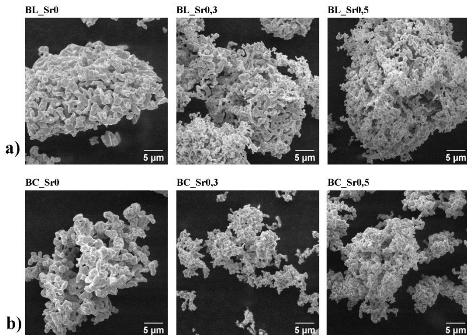
Slika 36. SEM mikrografije praškastih BSMO uzoraka pripremljenih (a) limunskim i (b) koprecipitacijskim postupkom sinteze, snimljene pri povećanju od 5000x.
