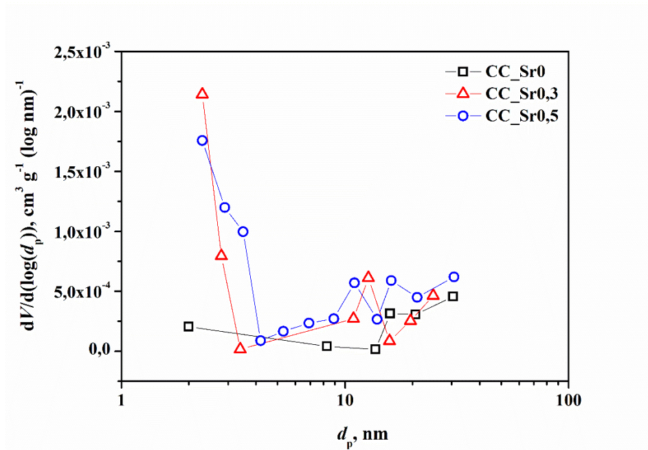
Slika 35. Raspodjela veličina pora CSMO uzoraka pripremljenih koprecipitacijskim postupkom sinteze.
