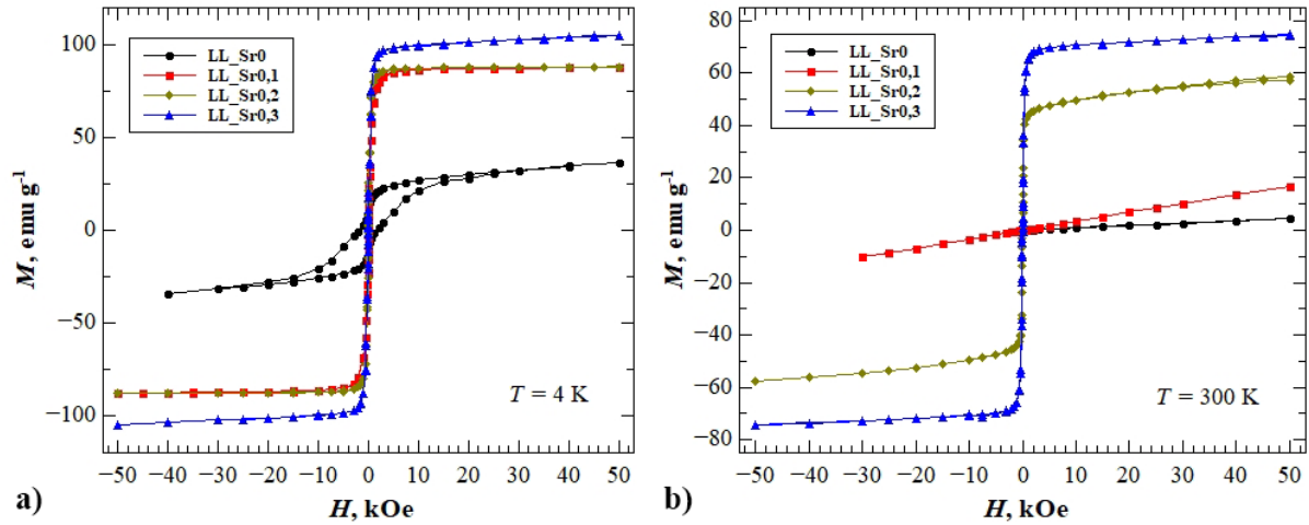
Slika 46. Magnetske histereze LSMO uzoraka pripremljenih limunskim postupkom sinteze snimljene pri temperaturama od (a) 4 K i (b) 300 K.
