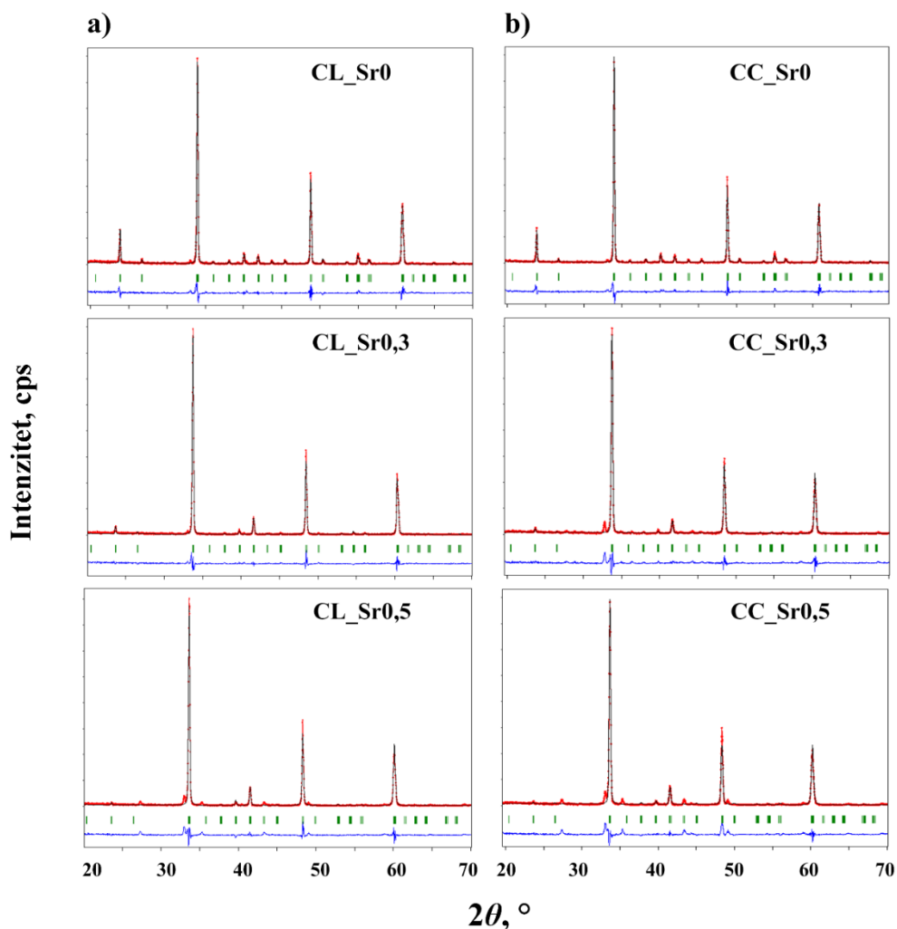
Slika 26. Rezultati Rietveldove metode utočnjavanja za CSMO uzorke pripremljene (a) limunskim i (b) koprecipitacijskim postupkom sinteze. Eksperimentalni podaci prikazani su crvenim točkama, izračunati model crnom linijom, a odstupanja eksperimentalnih podataka od modela prikazana su plavom linijom ispod difraktograma. Zelenim crtama prikazane su Braggeve pozicije za svaku od faza.
