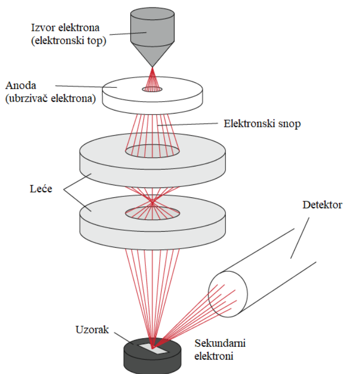
Slika 13. Shema pretražnog elektronskog mikroskopa [114].
