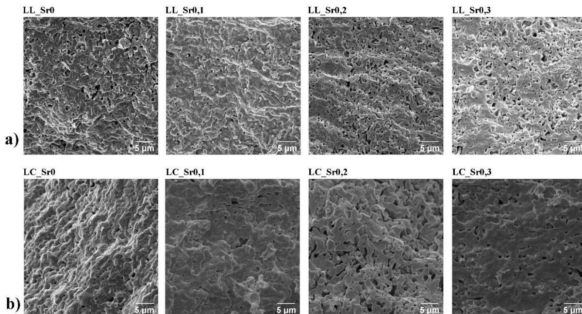
Slika 31. SEM mikrografije lomne površine LSMO peleta dobivenih iz prašaka pripremljenih (a) limunskim i (b) koprecipitacijskim postupkom sinteze, snimljene pri povećanju od 5000x.
