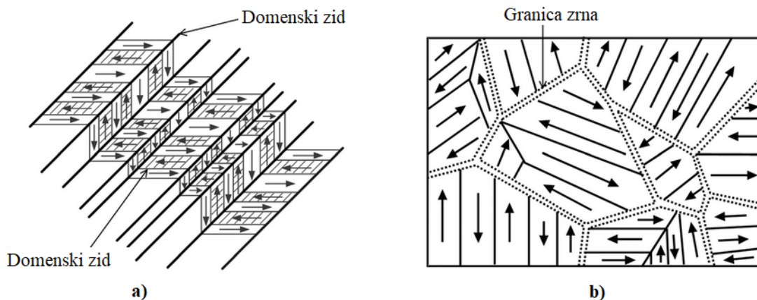
Slika 9. (a) Ilustracija pojma domenskih zidova i (b) primjer njihovog identificiranja TEM-om [80].
