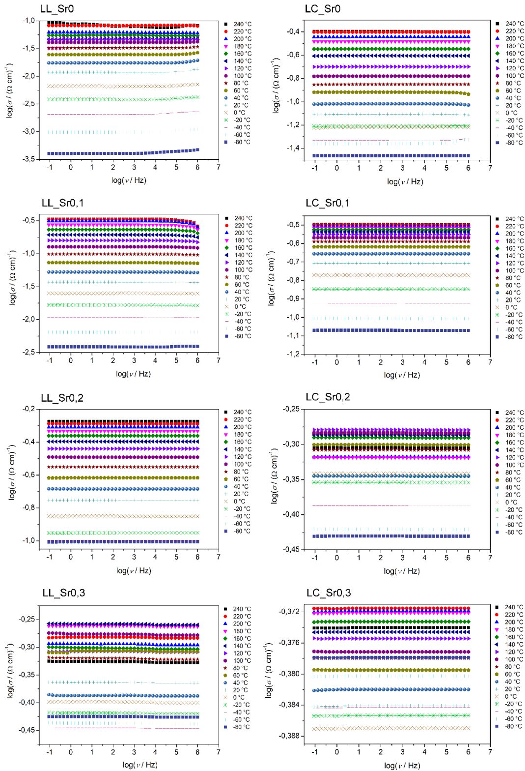
Slika P1. Frekvencijske ovisnosti električne provodnosti LSMO uzorka pripremljenih limunskim (oznake LL) i koprecipitacijskim (oznake LC) postupkom sinteze.
