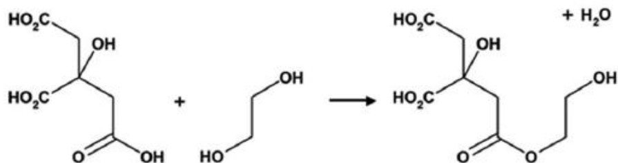
Slika 3. Reakcija transesterifikacije između limunske kiseline i etilen-glikola [42].
