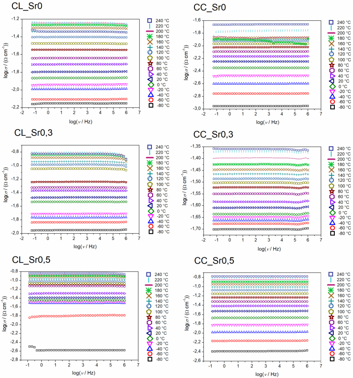
Slika P2. Frekvencijske ovisnosti električne provodnosti CSMO uzoraka pripremljenih limunskim (oznake CL) i koprecipitacijskim (oznake CC) postupkom sinteze.
