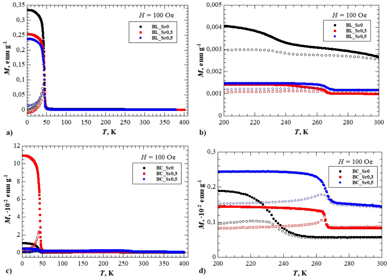
Slika 52. Magnetizacijske krivulje uzoraka BSMO pripremljenih limunskim (oznake BL, a i b) i koprecipitacijskim (oznake BC, c i d) postupkom sinteze izmjerene pri jakosti magnetskog polja od 100 Oe. Na slikama (b) i (d) dani su uvećani prikazi krivulja za dopirane uzorke. Šuplji simboli predstavljaju ZFC mjerenja, a ispunjeni FC mjerenja.
