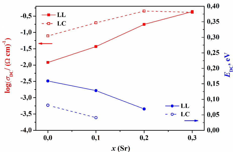
Slika 40. Ovisnosti istosmjernje provodnosti ( \sigma_{DC} ) na 20 °C i energije aktivacije ( E_{DC} ) o udjelu dopiranja LSMO uzoraka.
