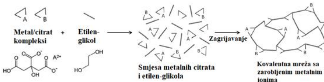
Slika 4. Shematski prikaz nastajanja kovalentne mreže sa zarobljenim metalnim ionima u Pechinijevoj metodi sinteze [42].
