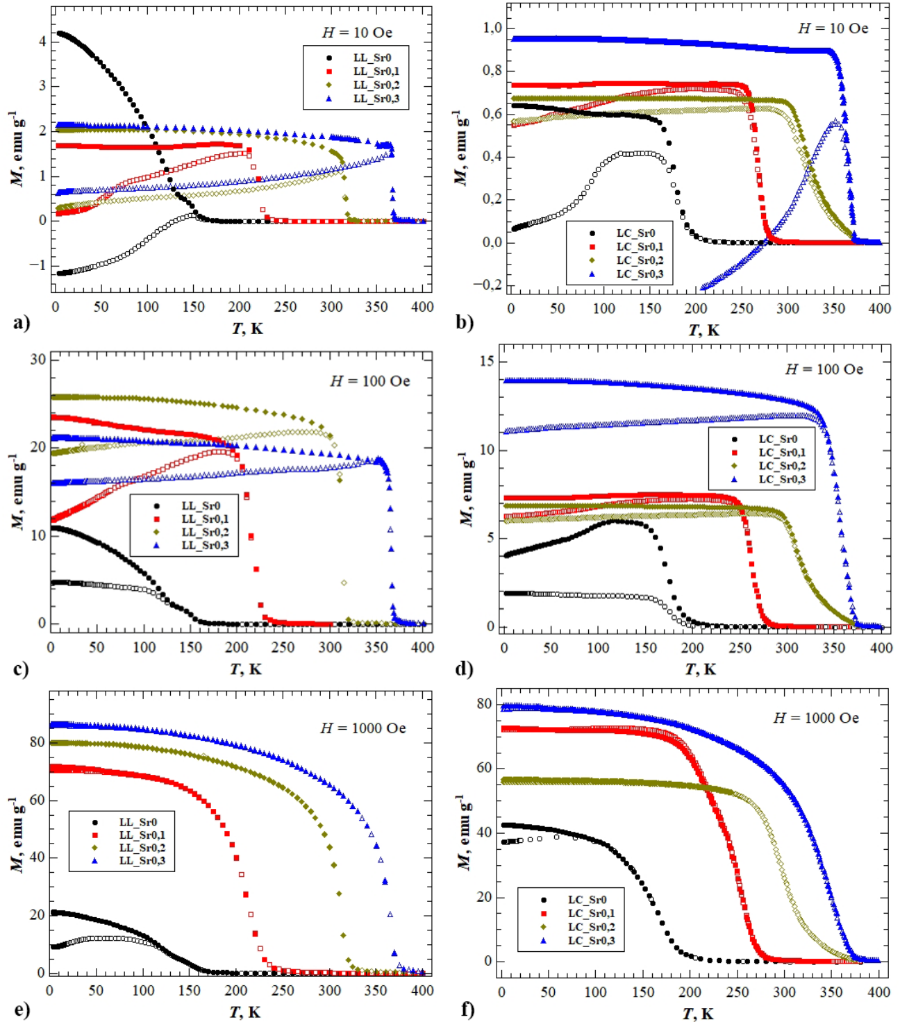
Slika 45. Magnetizacijske krivulje uzoraka LSMO pripremljenih limunskim (oznake LL, a, c i e) i koprecipitacijskim (oznake LC, b, d i f) postupkom sinteze izmjerene pri jakostima magnetskog polja od (a, b) 10 Oe, (c, d) 100 Oe i (e, f) 1000 Oe. Prazni simboli predstavljaju ZFC mjerenja, a ispunjeni FC mjerenja.
