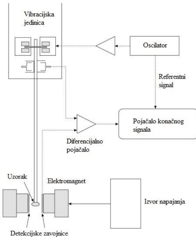
Slika 17. Shematski prikaz VSM magnetometra [121].
