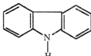
Karbazol
