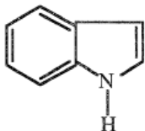
Indol
